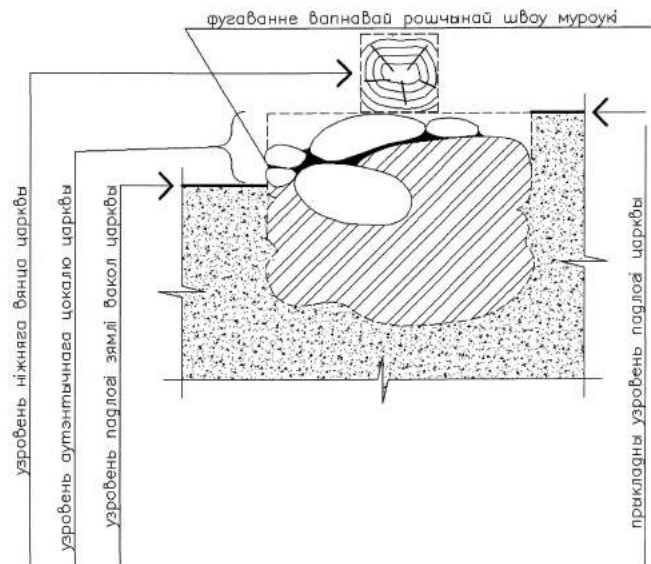
Іл. 21. Мікольская царква. Рэканструкцыя цокаля царквы
